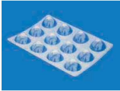
85112 12 Cell Lid, Fits #85113 O.D.: 7.000 x 5.250 x 0.625 I.D.: 1.375 x 1.375 x 0.500 Mat.: OPS, HIPS
