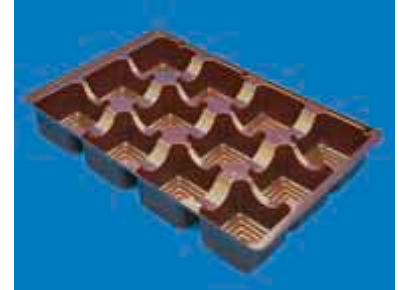
1312 12 Cell Tray O.D.: 9.375 x 6.000 x 1.000 I.D.: 1.625 x 1.625 x 1.000 Mat.: OPS, HIPS
