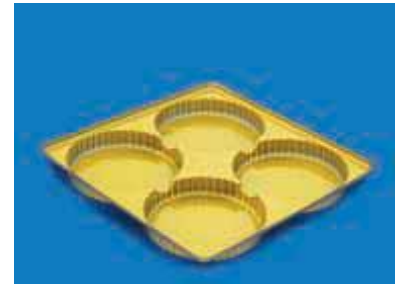
85104 4 Cell Tray O.D.: 6.125 x 6.125 x 0.625 I.D.: 2.750 x 2.750 x 0.625 Mat.: OPS, HIPS
