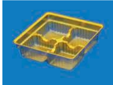
88750 4 Cell Tray O.D.: 3.875 x 3.875 x 1.000 I.D.: 1.500 x 1.500 x 1.000 Mat.: OPS, HIPS
