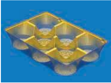
85108 8 Cell Tray O.D.: 6.250 x 4.250 x 1.250 I.D.: 1.500 x 1.500 x 1.250 Mat.: OPS, HIPS
