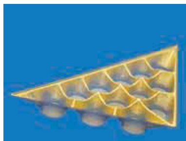
85122 12 Cell Triangle Tray O.D.: 9.375 x 9.875 x 1.250 I.D.: 1.500 x 1.500 x 1.250 Mat.: OPS, HIPS
